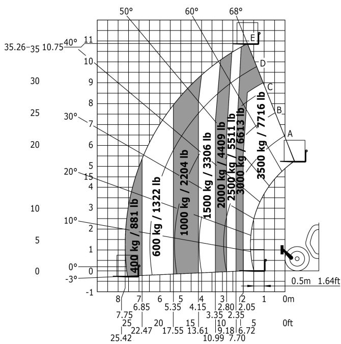
Macchina su pneumatici con forche
