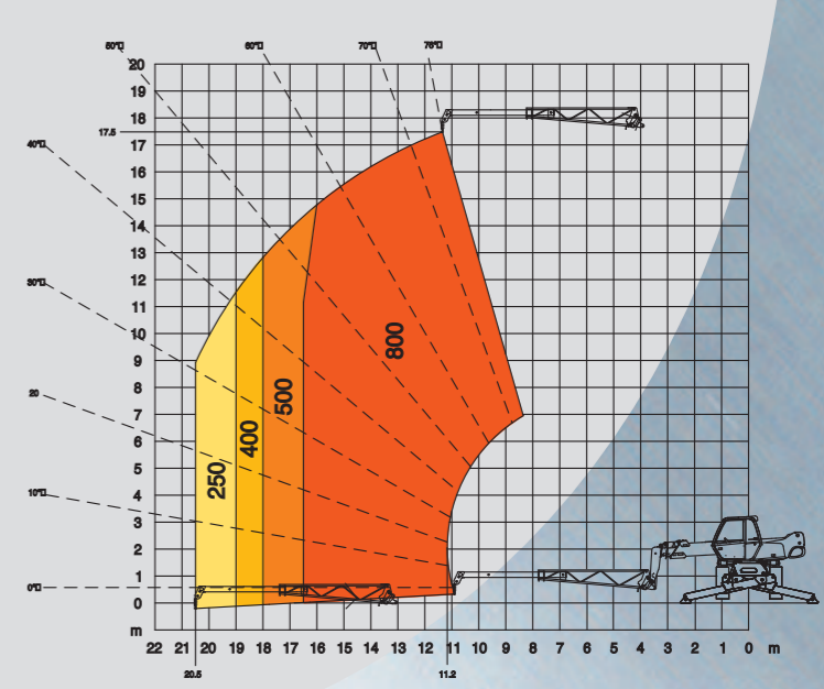
ROTAZIONE SU STABILIZZATORI COMPLETAMENTE SFILATI CON CRANE JIB
