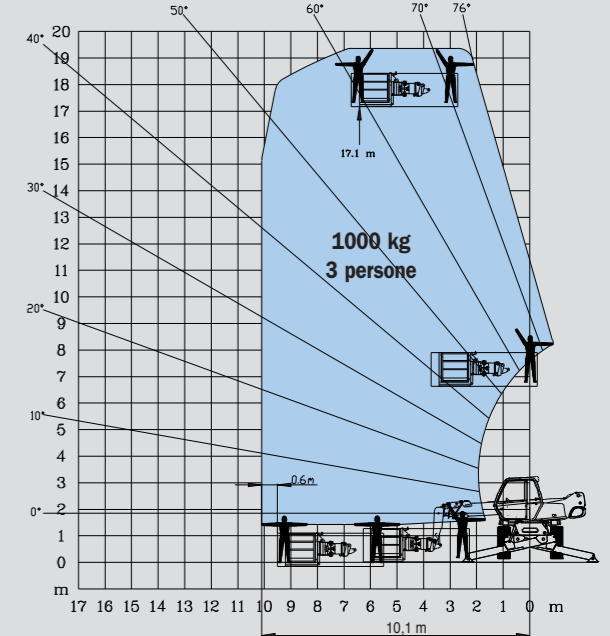
ROTAZIONE SU STABILIZZATORI COMPLETAMENTE SFILATI CON CESTELLO A PENDOLO ROTANTE 3 D LAVORO IN NEGATIVO
